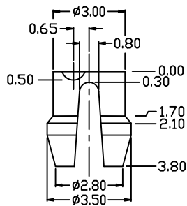
DETAIL Y
