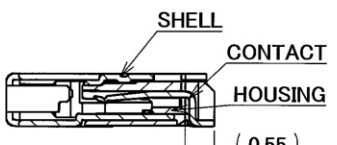
断面図 X-X スケール 10 : 1
