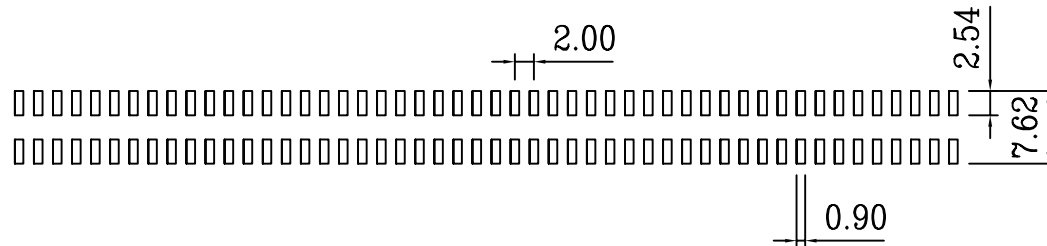
P.C.B.layout
