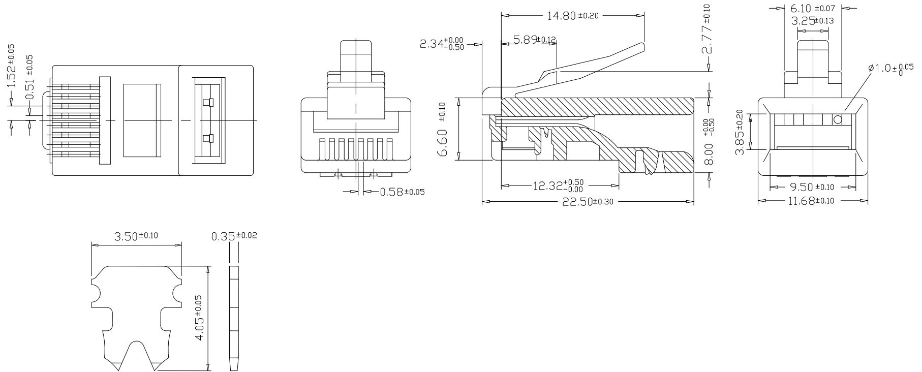
“ ” : PRONGS FOR STRANDED WIRE 多芯線用二叉型金片
