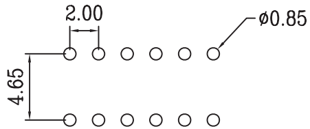
P.C.B.layout
