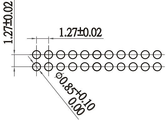
P.C.Board Layout
