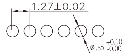
P.C.Board Layout
