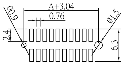
P.C.Board Layout
