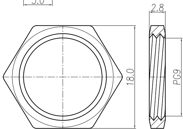
NUT
