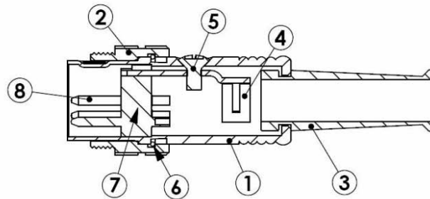
A-A SECTION
