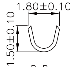
B-B
