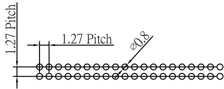
P.C.Board Layout
