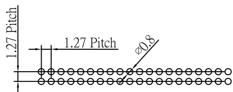
P.C.Board Layout
