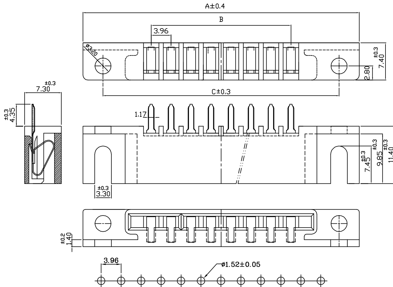
P.C.B LAYOUT
