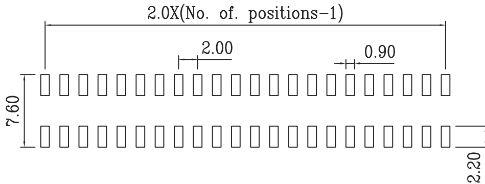
P.C.B. layout
