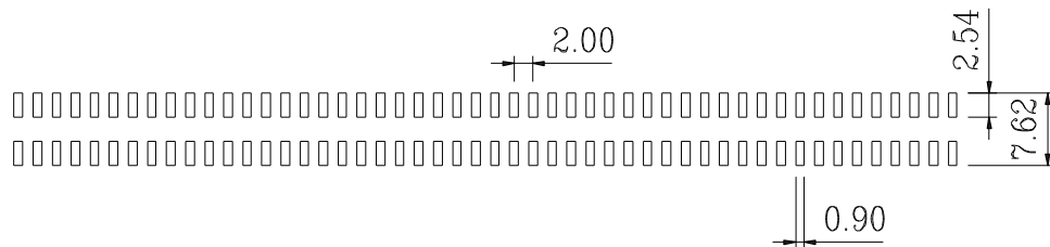
P.C.B.layout
