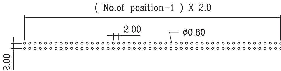
P.C.B.layout
