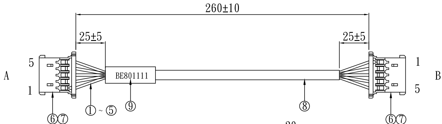
WIRING CHART
