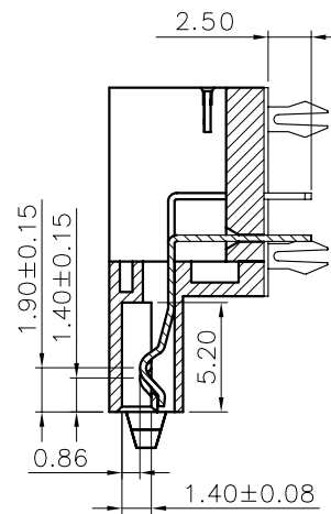
剖面圖 A-A 比例 1:1
