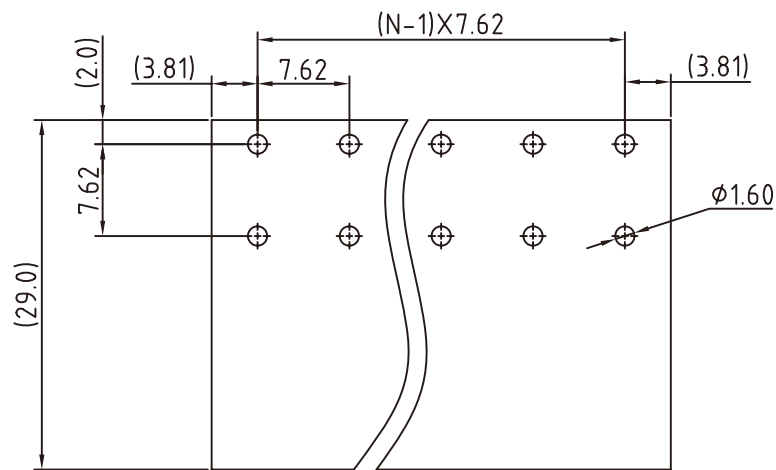
P.C.B LAYOUT
