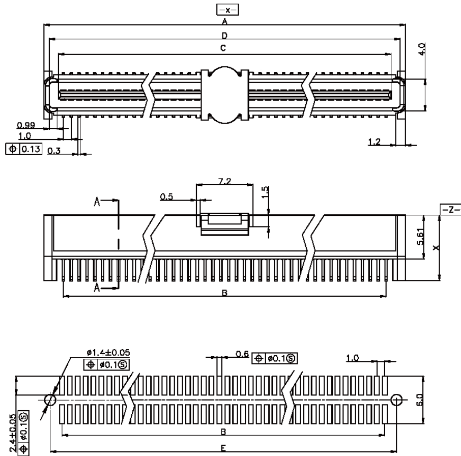
P.C.Board Layout
