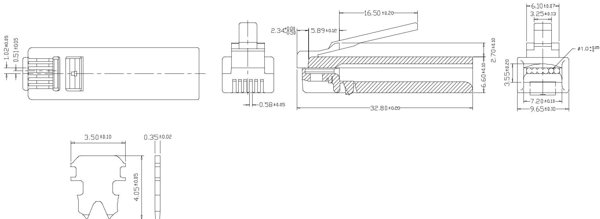
2 PRONGS FOR STRANDED WIRE 多芯線用二叉型金片
