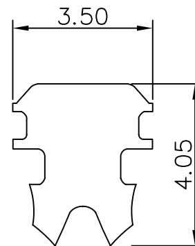
2 PRONGS FOR STRANDED WIRE 多芯線用二叉型金片
