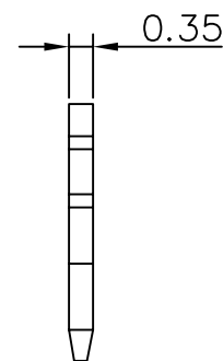
2 PRONGS FOR STRANDED WIRE 多芯線用二叉型金片
